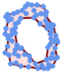
Forme alpha d'un MultiPoint, autorisant les trous (même exemple que ST_OptimalAlphaShape )
